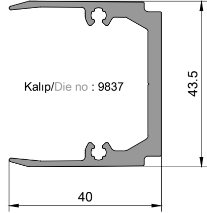
P 1425 YATAY MONTAJ PROFİLİ transom connector profile Ağırlık/Weight : 0,920 kg/mt
