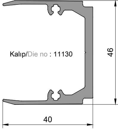
P 1424 YATAY MONTAJ PROFİLİ transom connector profile Ağırlık/Weight : 0,945 kg/mt
