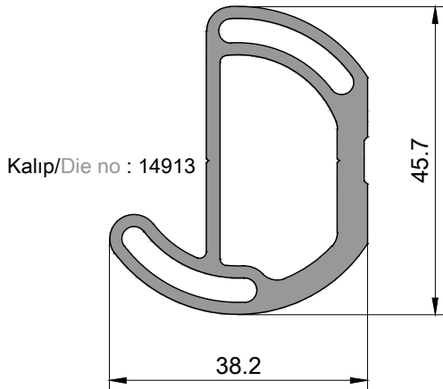
P 1426 AÇILI YATAY MONTAJ PROFİLİ angular transom connector profile Ağırlık/Weight : 1,140 kg/mt
