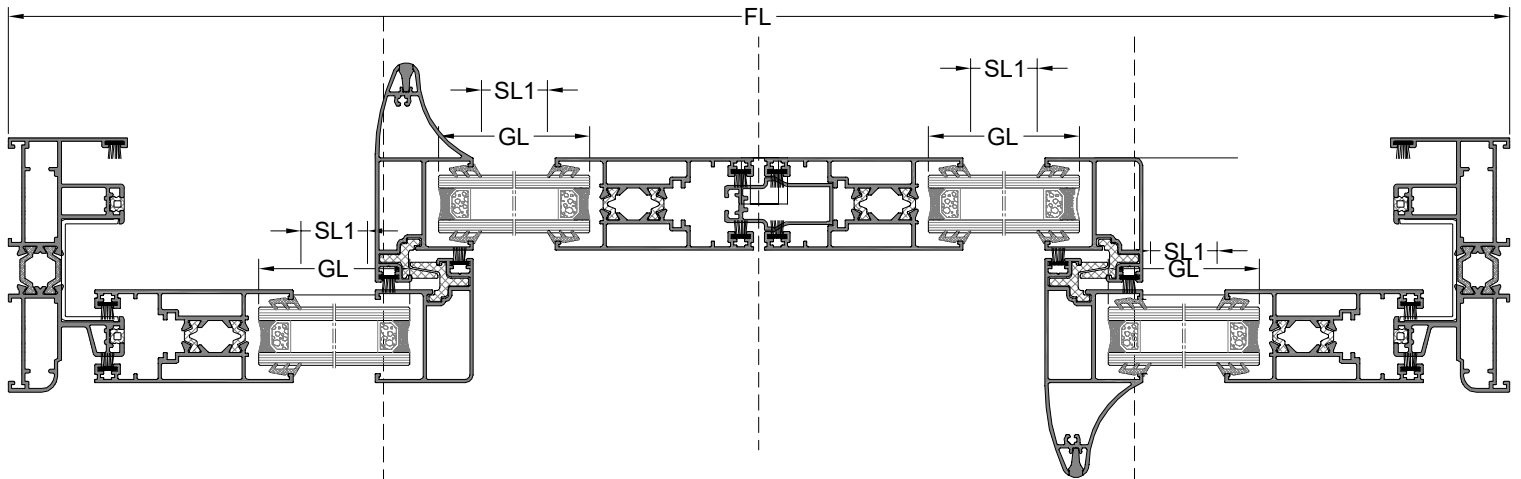
A-A KESİTİ
