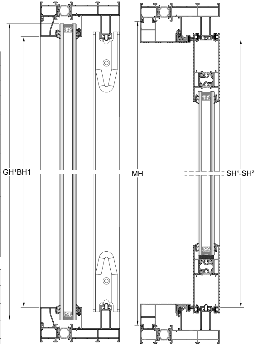
C-C KESİTİ
